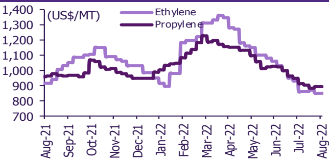
Olefins prices
