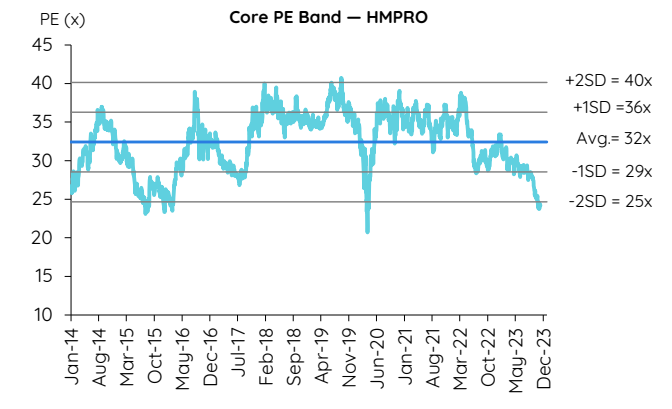
Figure 6: Historical core PE band สำหรับ HMPRO
