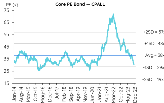
Figure 3: Historical core PE band สำหรับ CPALL
