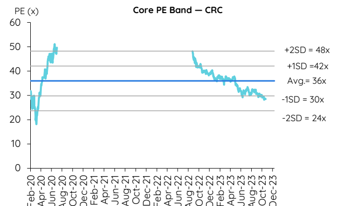
Figure 8: Historical core PE band สำหรับ CRC
