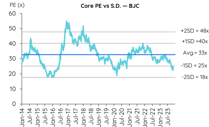
Figure 5: Historical core PE band สำหรับ BJC
