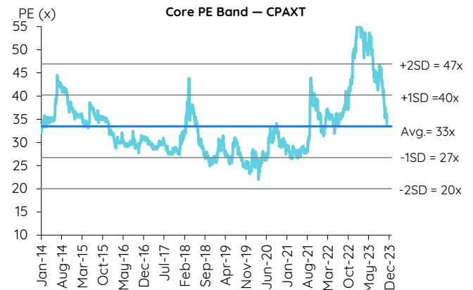
Figure 4: Historical core PE band สำหรับ CPAXT
