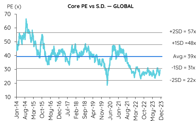
Figure 7: Historical core PE band สำหรับ GLOBAL
