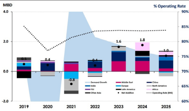
Figure 15: การเพิ่ม CDU ทั่วโลก VS อุปสงค์เพิ่มเติม
