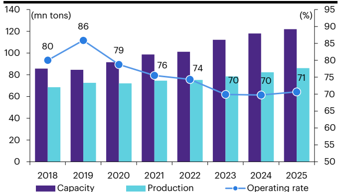
Figure 45: กำลังการผลิตและอัตราการใช้งาน PTA ทั่วโลก
