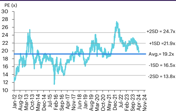
Figure 8: PE Band
