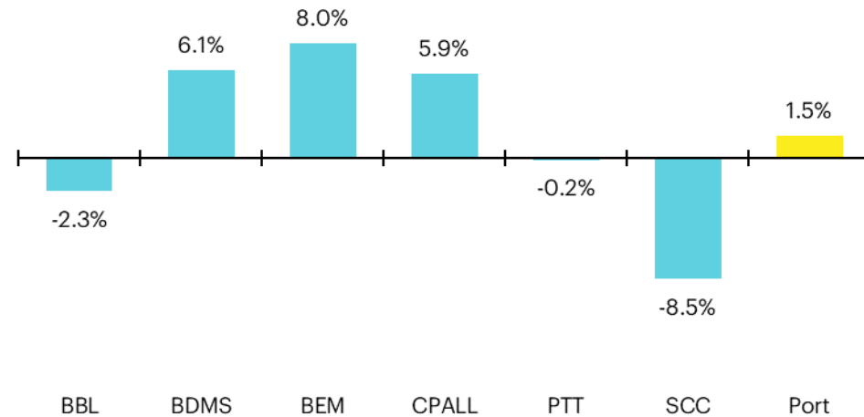
ผลการดำเนินงานสะสมของหุ้นและพอร์ต (30 พ.ย. 23 - 30 เม.ย. 24)
