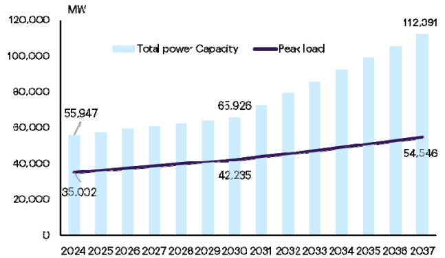
Figure 2: PDP 2024: กำลังการผลิตไฟฟ้าสุทธิ และ peak load ในปี 2567-2580
